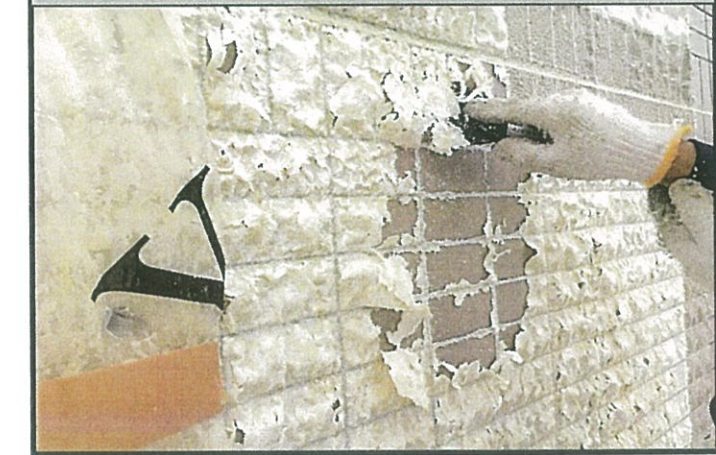
⑧その後、残存塗膜を※カーボンヘラで剥がしていく。 タイル面に限り金属ヘラは使用しない事。 (タイル表面が黒ずんでしまう為)
