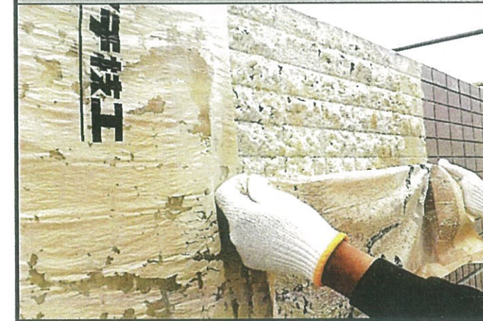
⑦YGシートをゆっくり剥がしていく。 (旧塗膜の劣化度によってシートに転写されて一緒に剥がれる場合がある)
