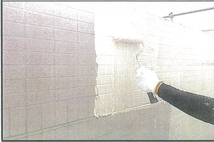
②ハーガスNEOをループローラーで1.0kg/㎡以上塗布する。 ※塗布量が規定量に満たない場合、
